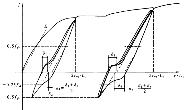
图 A.0.1-3 大变形反复拉压
