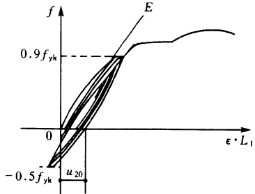
图 A.0.1-2 高应力反复拉压
