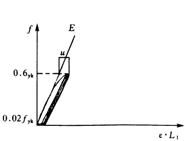
图 A.0.1-1 单向拉伸
