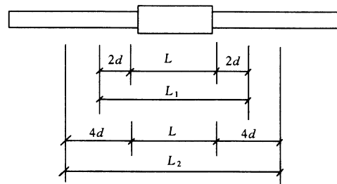
图 5.0.3 接头试件变形测量标距
